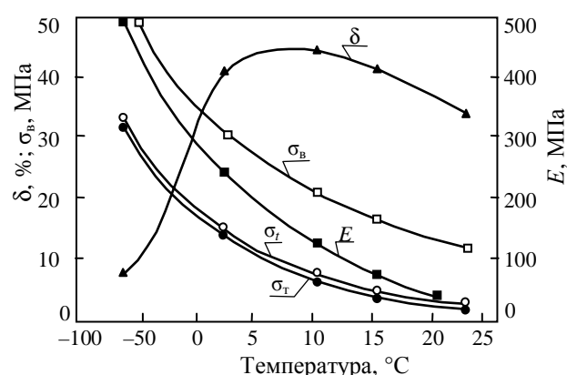
Рис. 1. Температурная зависимость прочности \sigma_{\text{в}} , предела текучести \sigma_{\text{т}} , модуля упругости E , относительного удлинения при разрыве \delta при растяжении фторопластовых трубок и разрушающего тангенциального напряжения \sigma_{\text{т}} (испытания под давлением)
