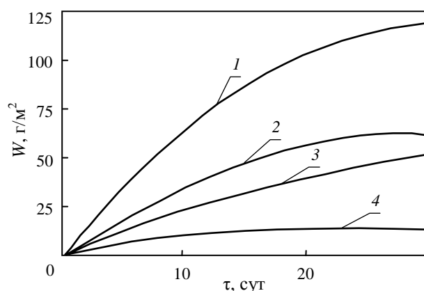
Рис. 2. Зависимость влагонабухания W стеклопластика на феноло-фурфурольном связующем от продолжительности увлажнения \tau .
